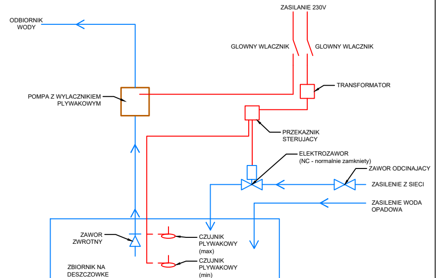
SCHEMAT INSTALACJI (OPCJA 2):
