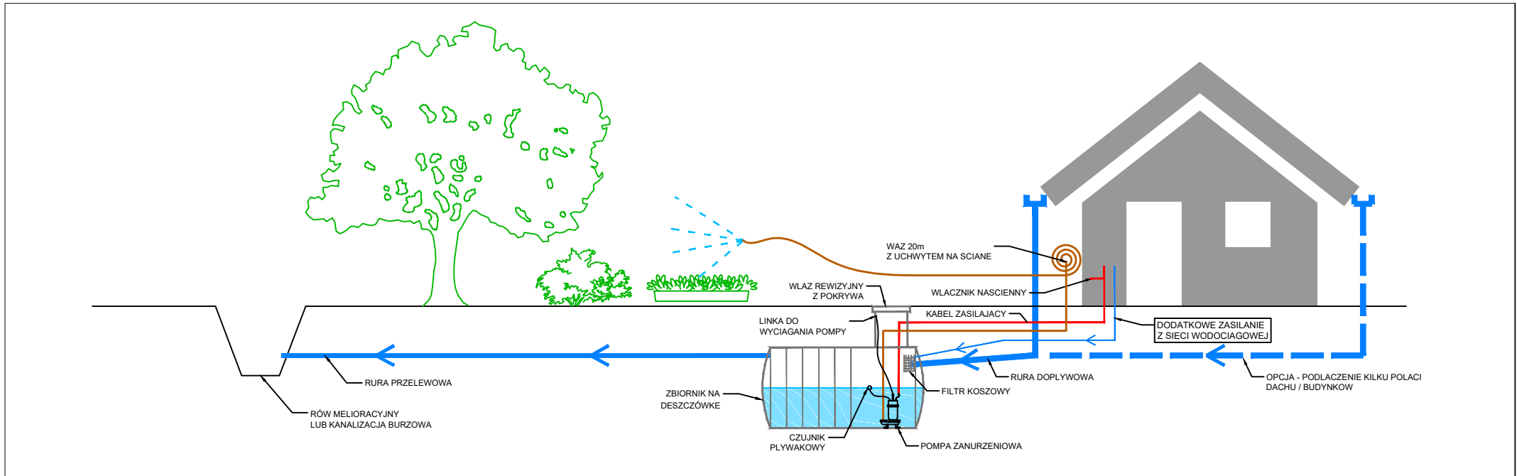
SCHEMAT INSTALACJI (OPCJA 2):
